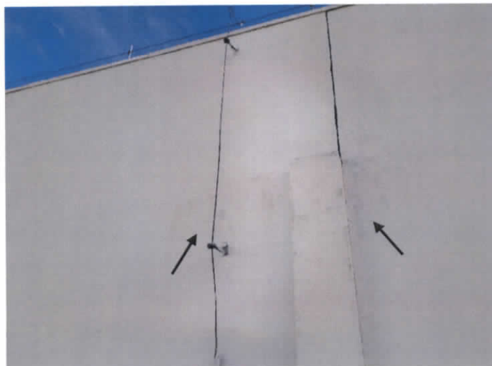
Foto 17 – Fachada externa em frete ao estacionamento Data: 24 de janeiro de 2017
