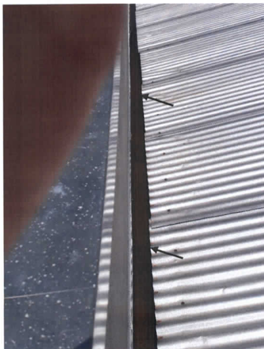
Foto 28 – Acumulo de água da chuva na calha Data: 24 de janeiro de 2017
